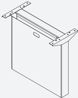
Detalhe pés
